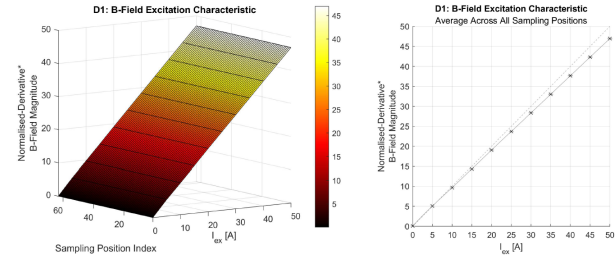
Figura 1: Non-linearitatea caracteristicii de excitatie. Caracteristica liniara in limita I_{ex} \leq 12\text{ A}
